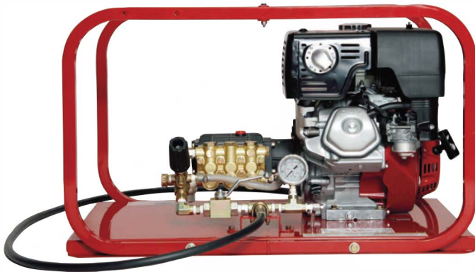
TRH-8 · 4 GPM · 3600 PSI
