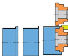
F6 Necking rolls
